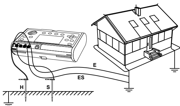
El sistema de medición de la impedancia de puesta a tierra (método de impulso 4p)
